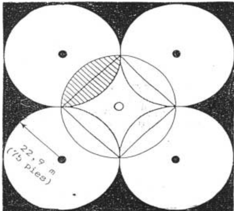
FIGURA 3 – Área cuadrada que representa el área máxima (1045 m 2 ) que el extintor puede proteger dentro de los límites de un radio de 22.9
